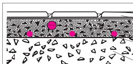
Рис.5. Тонкий пол на существующем бетонном полу.
