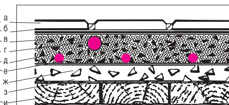
Рис.6. Тонкий пол на существующем деревянном полу.
